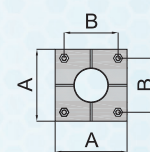
DETALHE POSTE FLANGEADO
